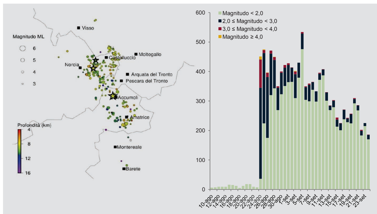
Figura 1.4 Eventi sismici in Italia centrale per classe di magnitudo Agosto-Settembre 2016, numero di eventi
